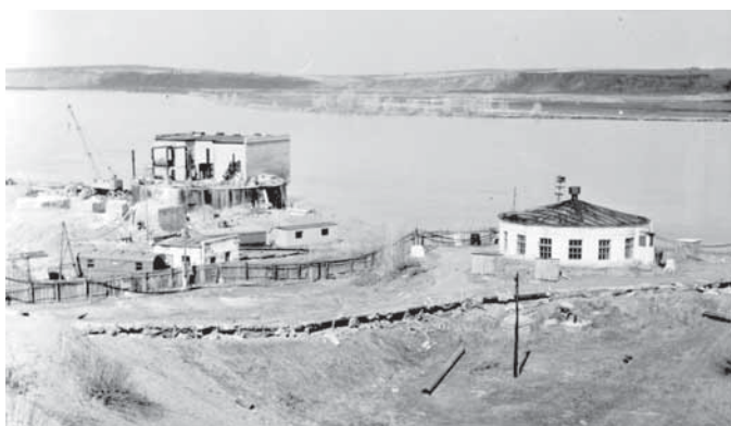
На фото: идет строительство насосной станции первого подъема и ковшевого водозабора, 1977 год. Фото из архива ОАО «КемВод».
