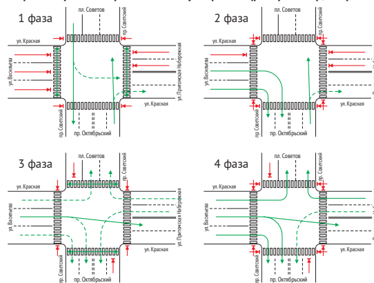
Пофазный разезд пр. Советский – ул. Красная (реверс вечер, + стрелка)
