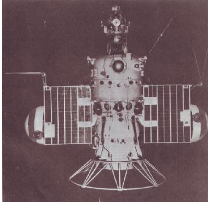
Автоматическая межпланетная станция «Марс-1».
